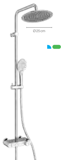
A 2 Atrio termostático Ref. ACOND120B sin IVA 383,50 € Altura: 120 cm Cartucho termostático Vernet. Rociador de acero inox., 25 cm Flexo de PVC plateado, teleducha de 3 posiciones y soporte regulable en altura. Derivador integrado en el cuerpo del grifo accionado por botones.
